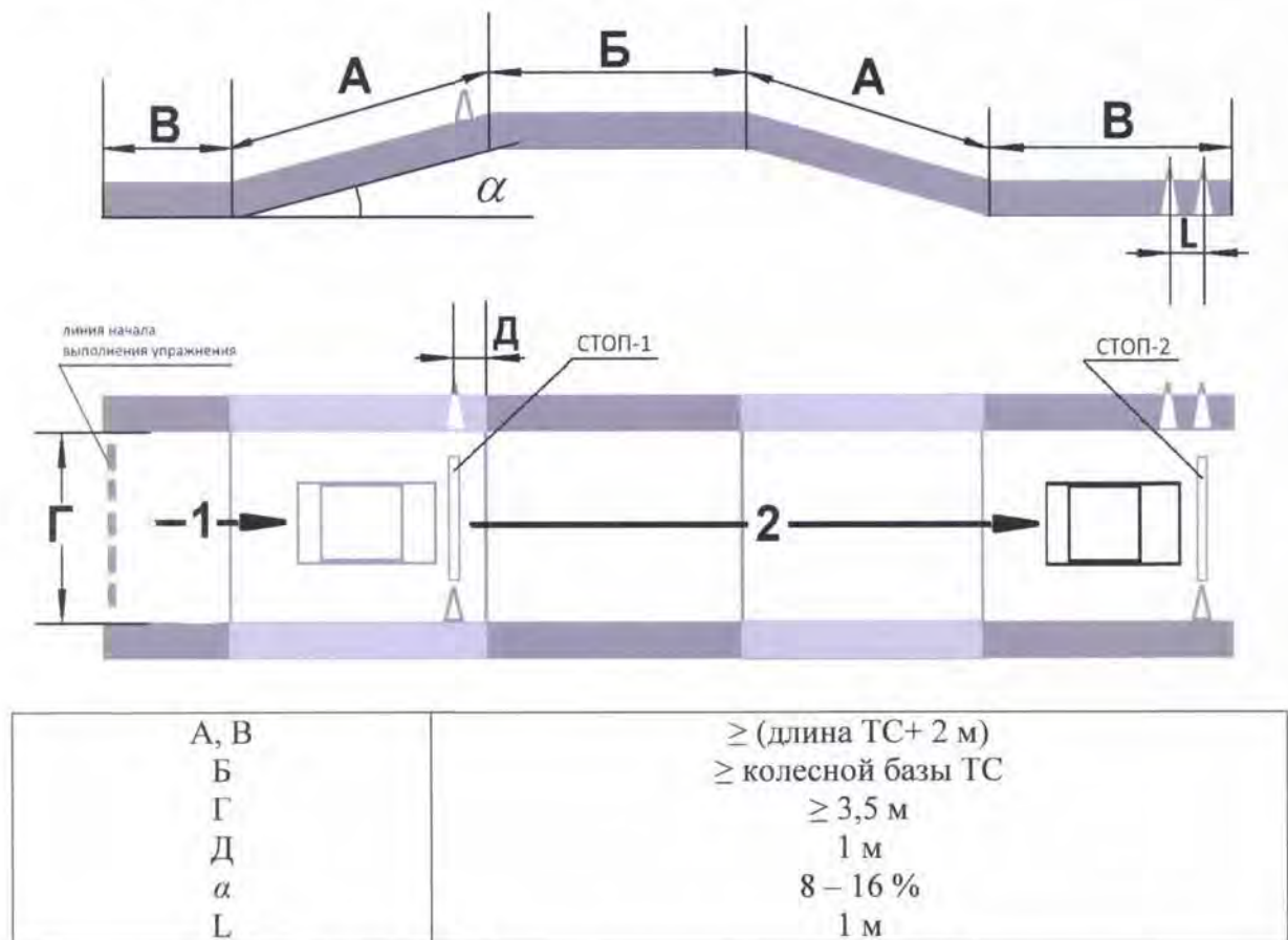
Рисунок 7. Схема и размеры упражнения № 4
