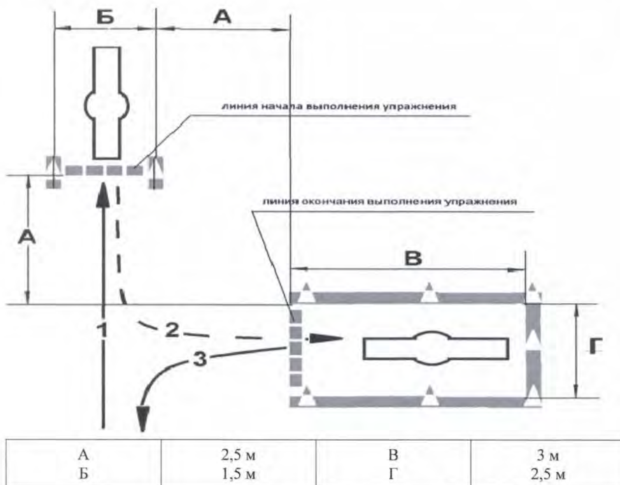
Рисунок 5. Схема и размеры упражнения № 2
